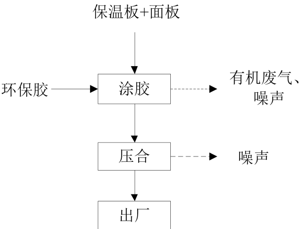
图 5-1 营运期工艺流程及产污图
