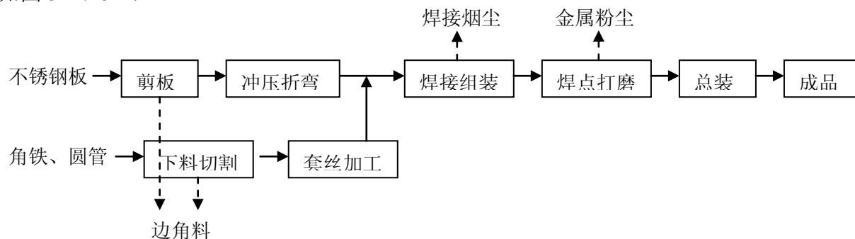
图 5-1 不锈钢成套厨房设备、商用燃气灶具生产工艺流程与产污图
