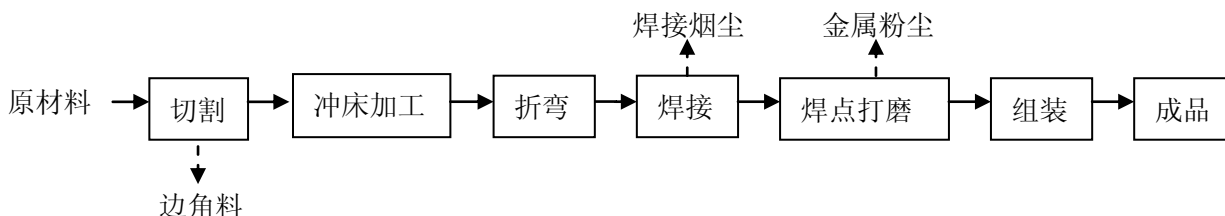
图 5-1 生产工艺流程与产污图
