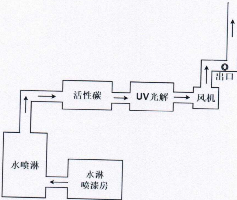
有组织废气检测流程示意图：
