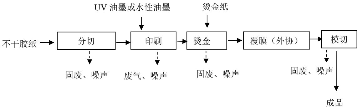
图 5-1 项目工艺流程图
