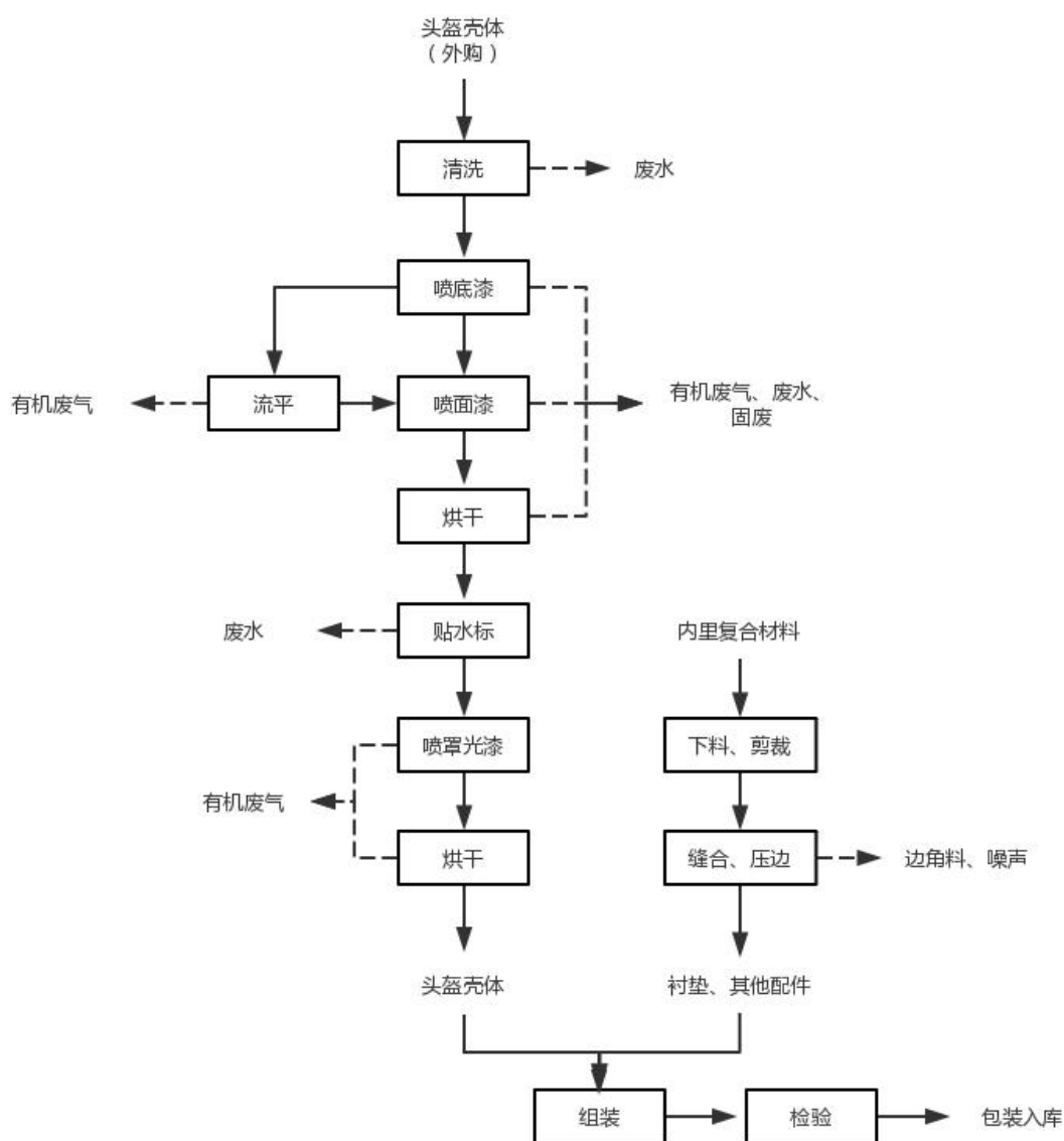
图 5-1 项目工艺流程及产排污节点示意图
