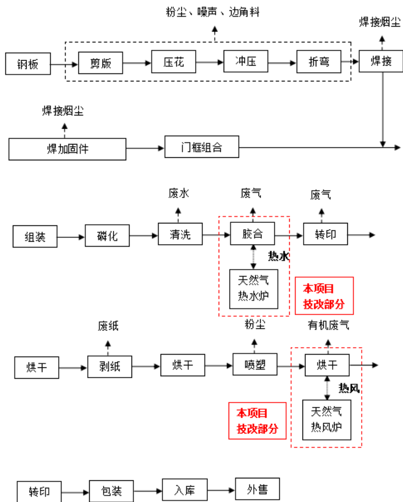
图 7-1 技改项目建成后全厂生产工艺流程及产污环节图
