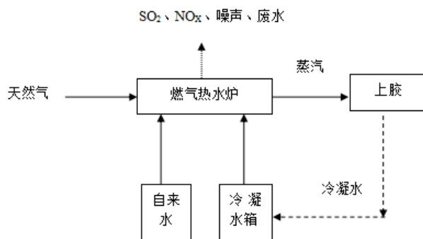
图 7-2 天然气热水炉生产工艺流程及产污环节图
