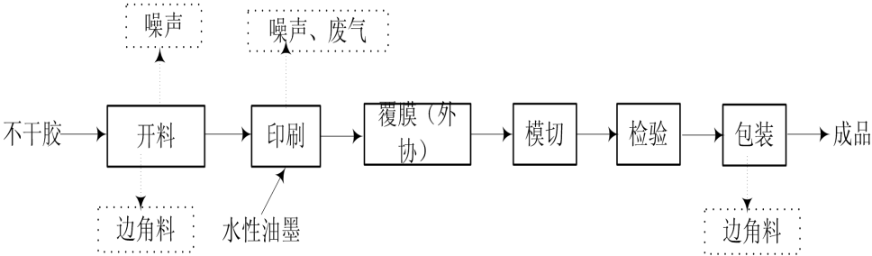
图 2-2 不干胶生产工艺及产污节点示意图
