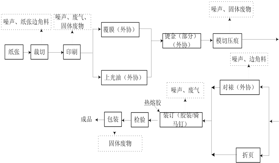
图 2-1 册子生产工艺及产污节点示意图
