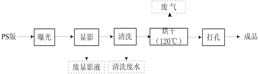
图 2-6 制版工艺及产污节点示意图
