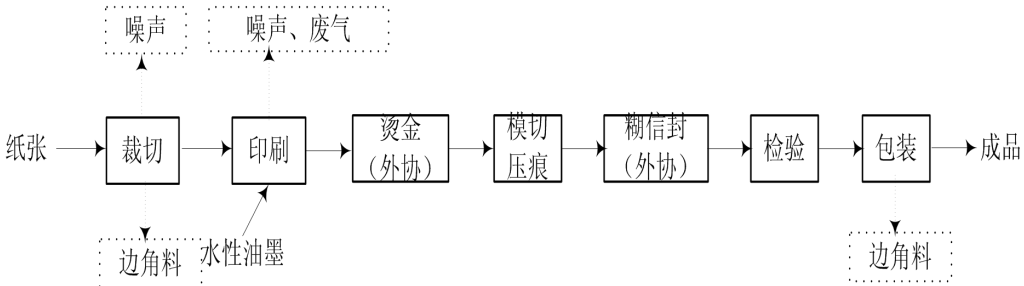
(3) 信封生产工艺及产污节点示意图
