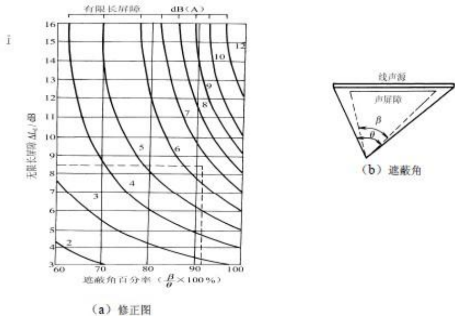
图 7-2 有限长度的声屏障及声源的修正图
