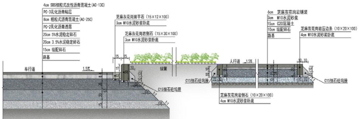
图 1-4 道路结构设计图
