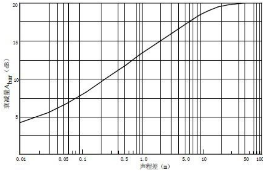
图 7-4 噪声衰减量 A_{\bar{a}} 与声程差 \delta 关系曲线 ( f=500\text{Hz} )
