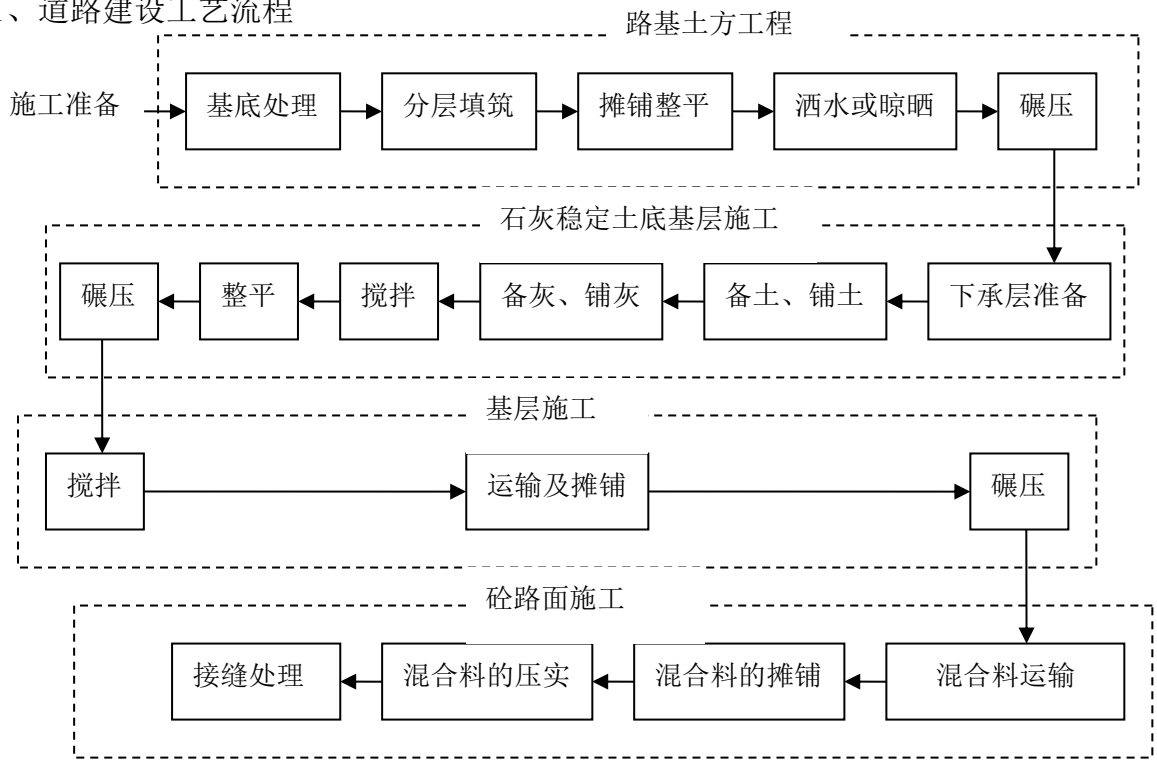
图 5-1 项目主要工程活动及产物节点图
