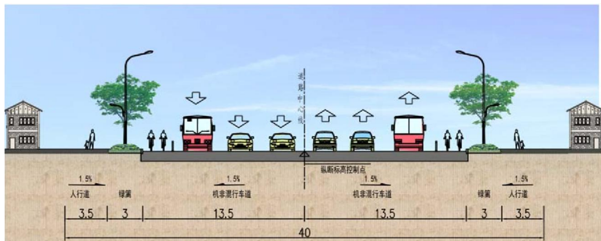
图 1-3 道路横断面图
