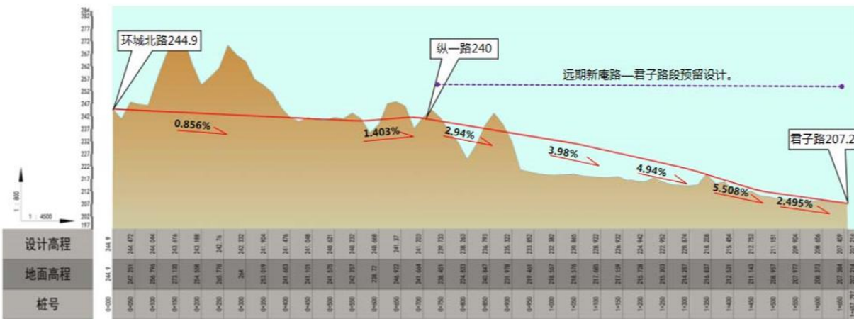
图 1-2 纵一路纵断面图
