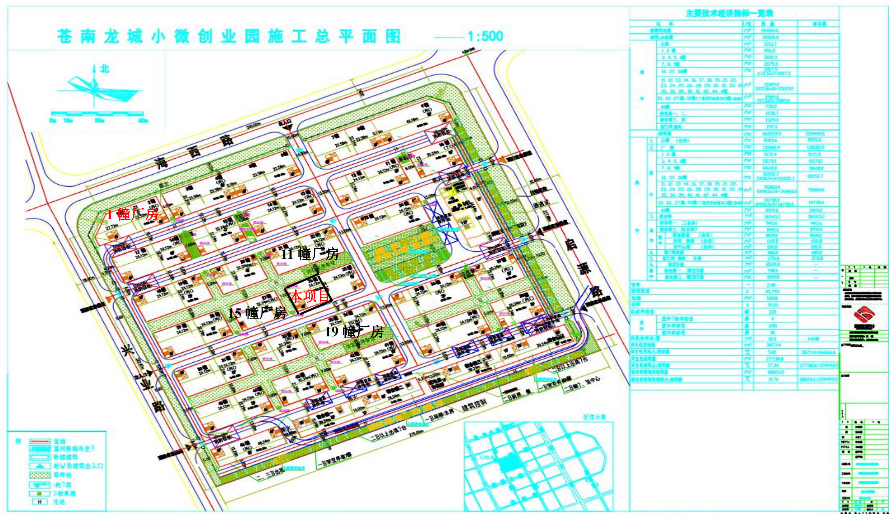
附图八 龙港龙诚小微创业园总平图
