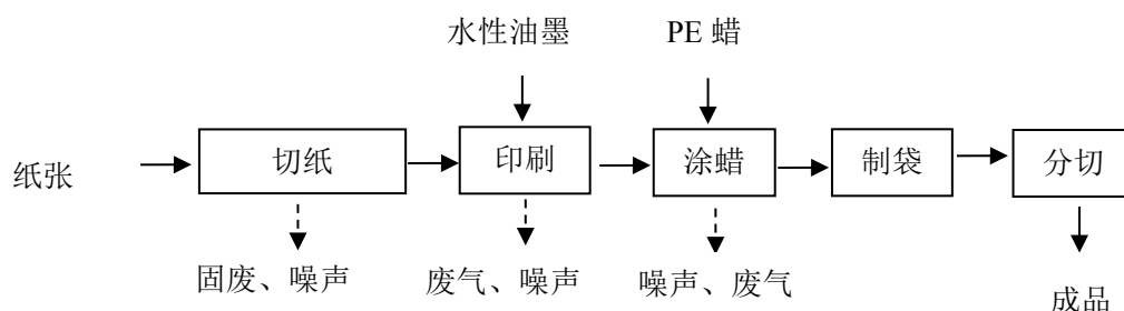
食品包装袋生产工艺流程图
