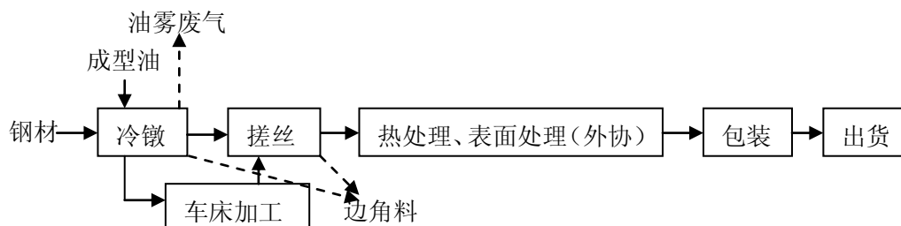
图 5-1 生产工艺流程及产污图
