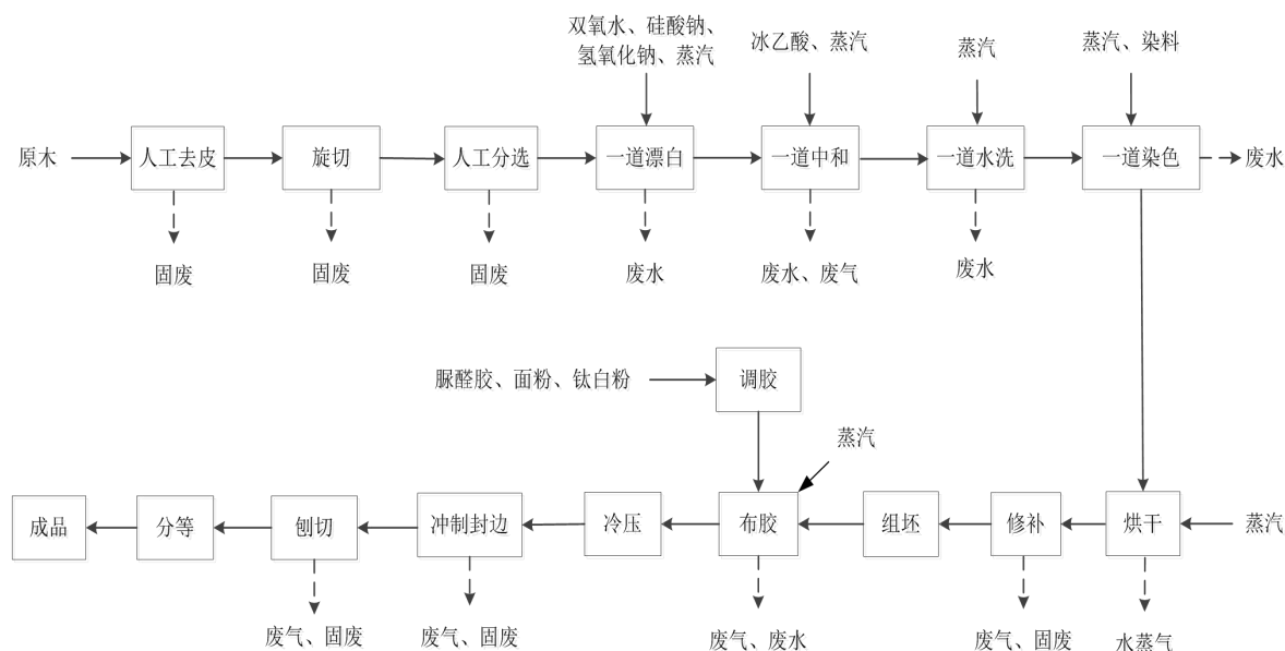
图 1-1 重组装饰材生产工艺流程图
