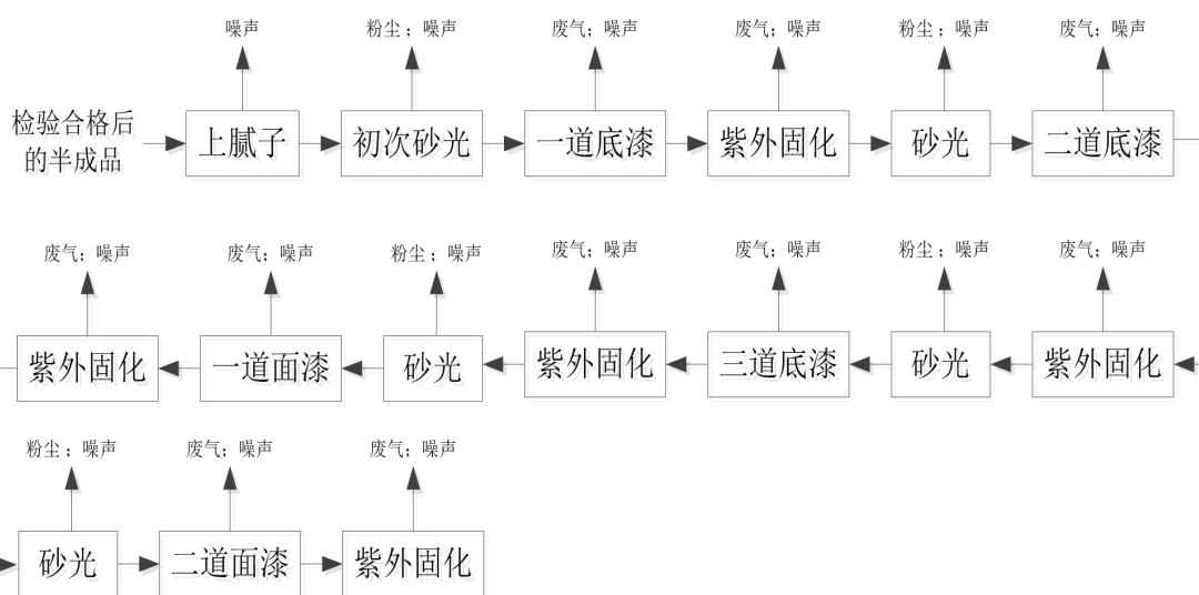
图 5-3 UV 辊涂工艺流程及产污环节示意图
