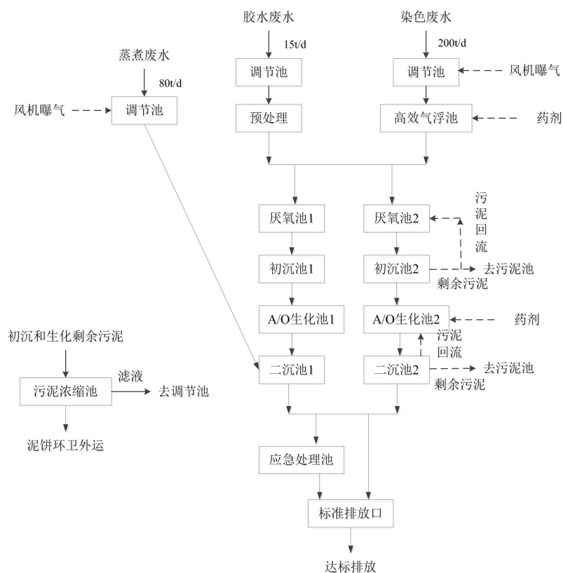
图 5-4 企业自建污水站工艺流程图
