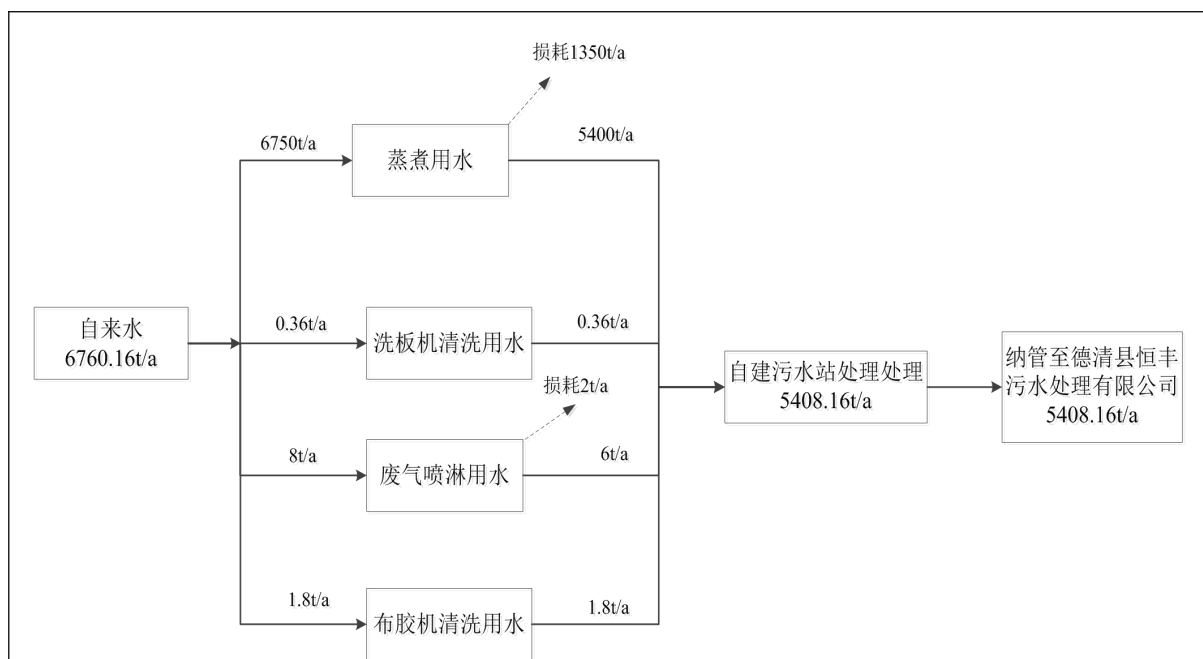
图 5-5 本项目水平衡图
