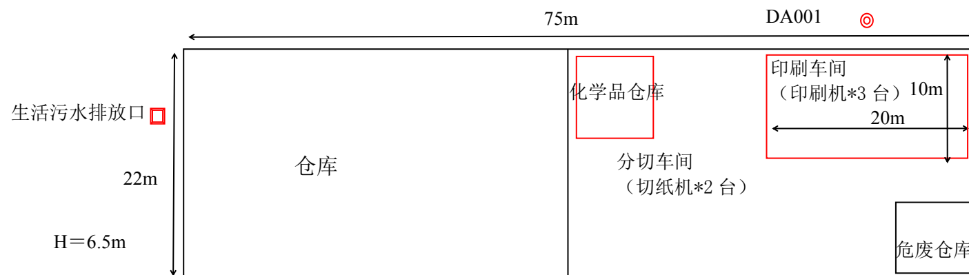
生产车间一层布置图
