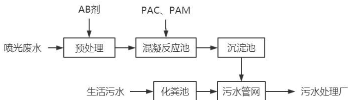
图7-1 本项目废水处理工艺流程图
