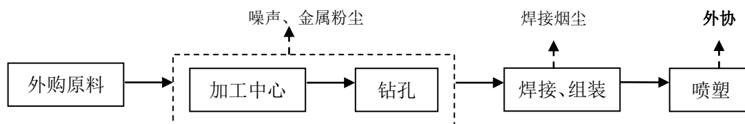
图 5-1 机壳生产工艺流程及产污环节
