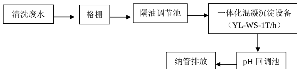
图 7-1 清洗废水处理流程图
