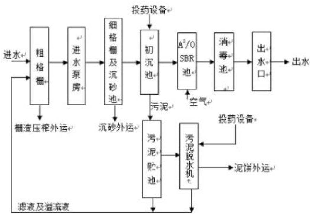
图 2-1 缙云县壶镇污水处理厂处理工艺流程图
