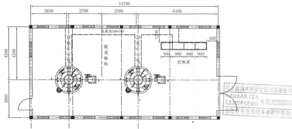
控制屏、电缆沟平面
