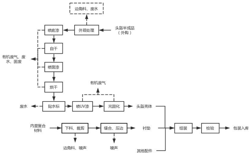
图 5-1 项目工艺流程及产排污节点示意图
