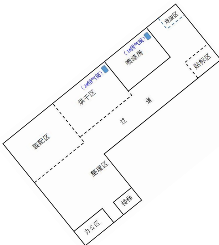
图 1-3 项目车间平面布置图
