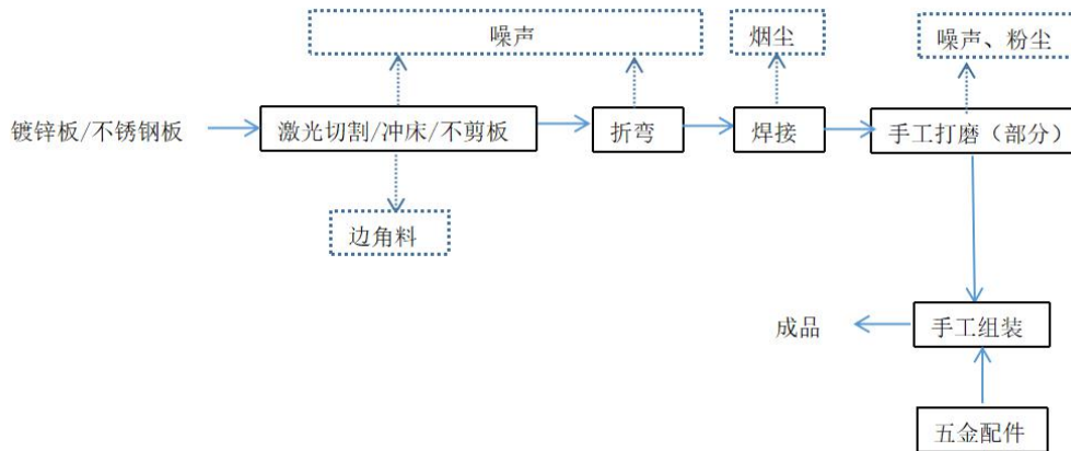
图 5-1 项目生产工艺流程及产污点图
