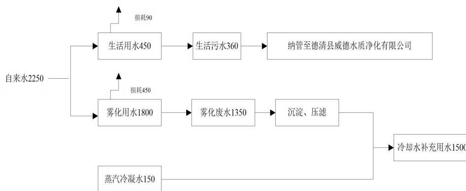
图 5-2 水平衡图
