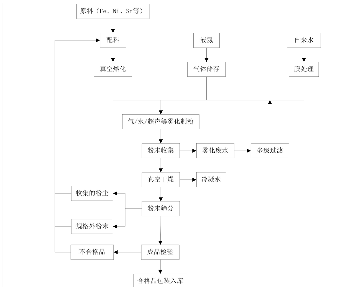
图 1-1 金属粉末生产工艺流程图（噪声伴随整个工艺）
