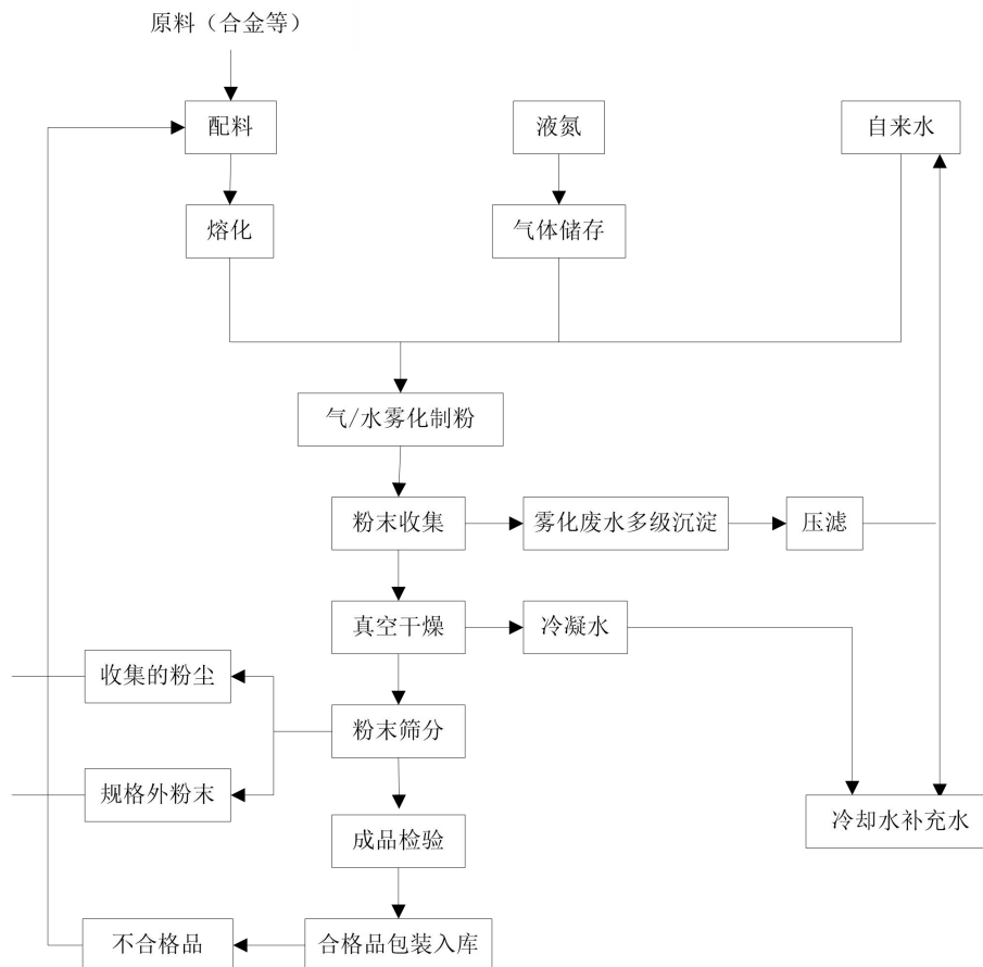
图 5-1 金属粉末生产工艺流程及产污节点图（噪声伴随整个工艺）
