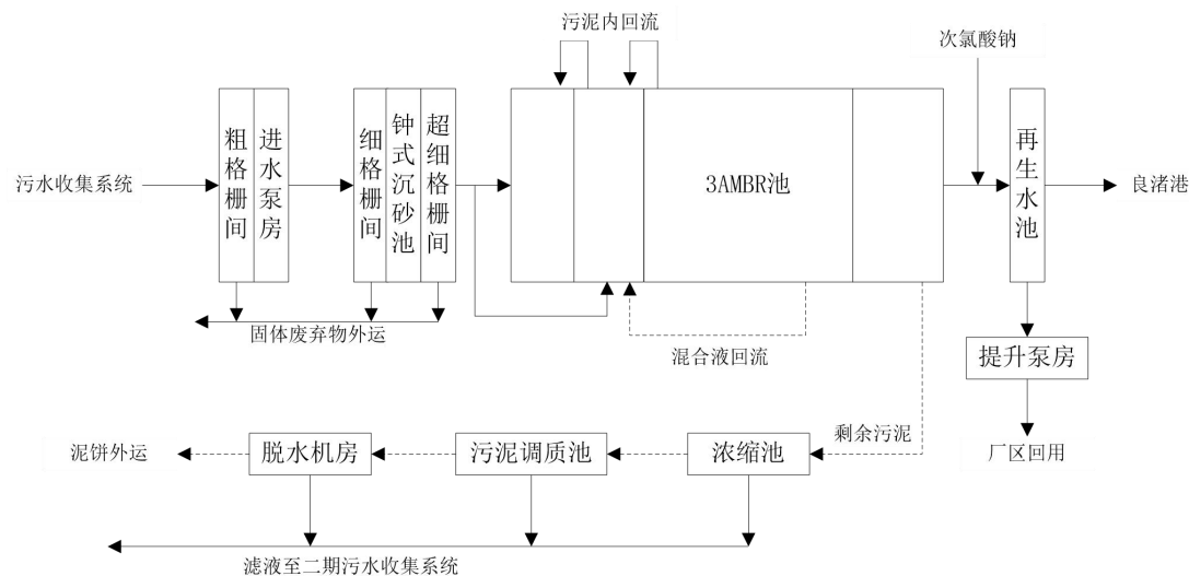
图 2-2 良渚污水处理厂三期工程实际污水处理工艺流程图
