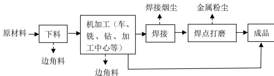
图 5-1 生产工艺流程与产污图
