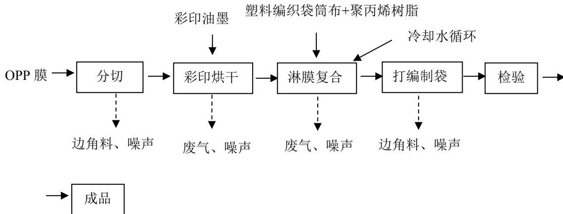
图 5-1 项目工艺流程图
