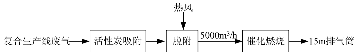
图 8-1 废气处理工艺流程图
