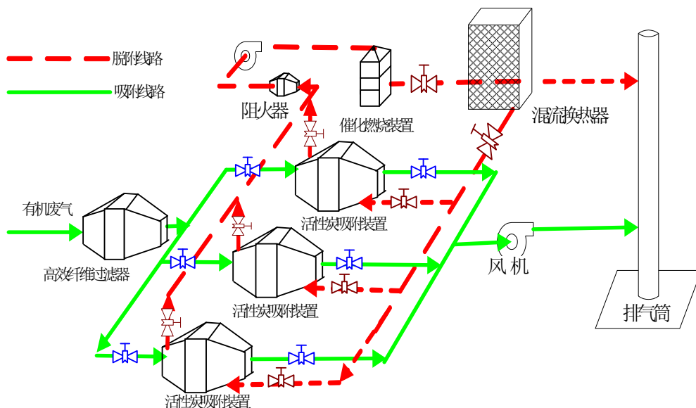
图 8-2 活性炭吸附浓缩+催化燃烧装置处理工艺流程图
