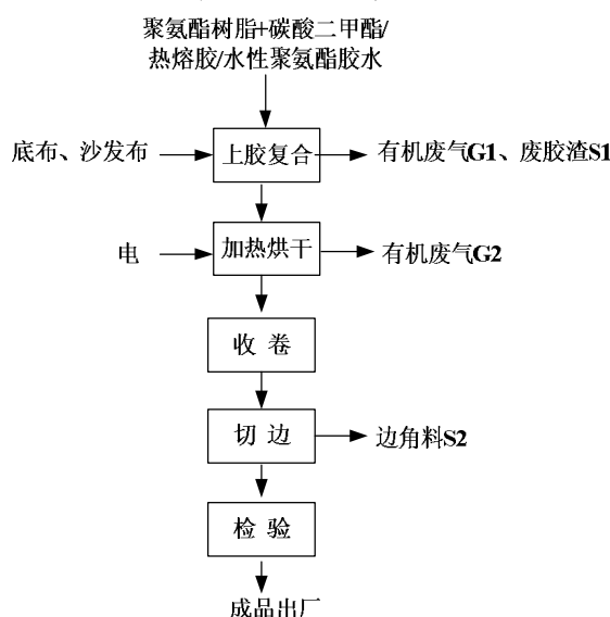
图 5-1 本项目生产工艺及产污环节图
