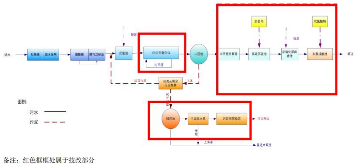
图2-1 乐清市污水处理厂处理工艺流程图
