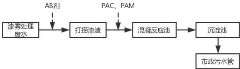
图 7-1 废水处理设施工艺流程图
