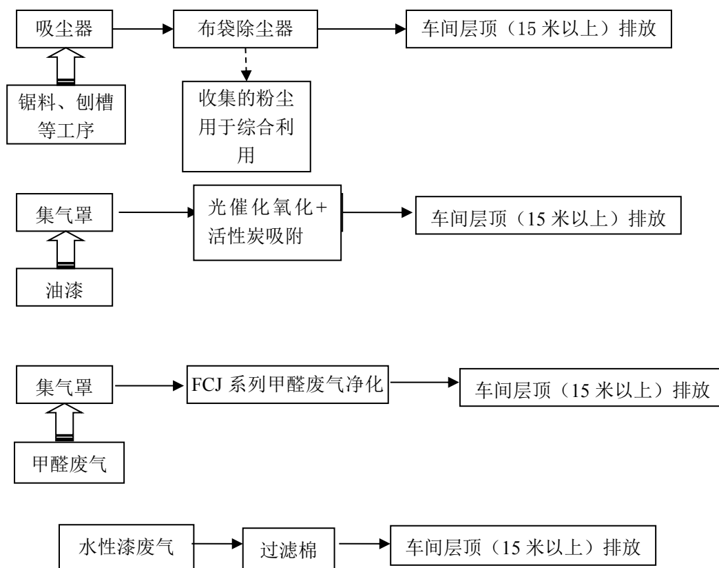
图 5-3 工艺废气治理流程图
