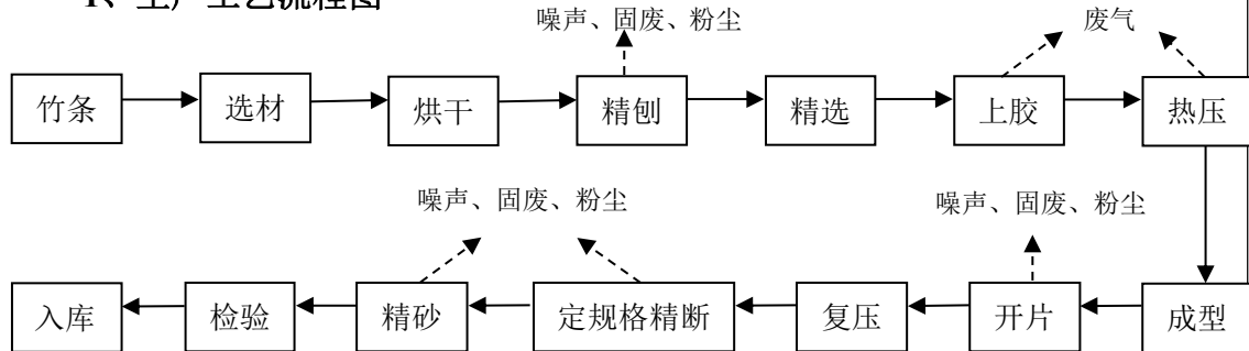
图 5-1 竹板材生产工艺
