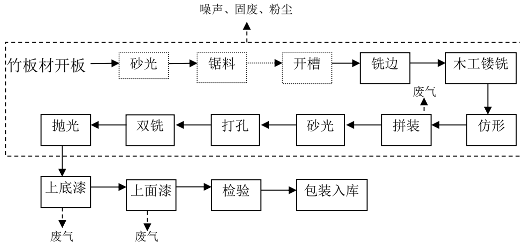
图 5-2 小家具生产工艺
