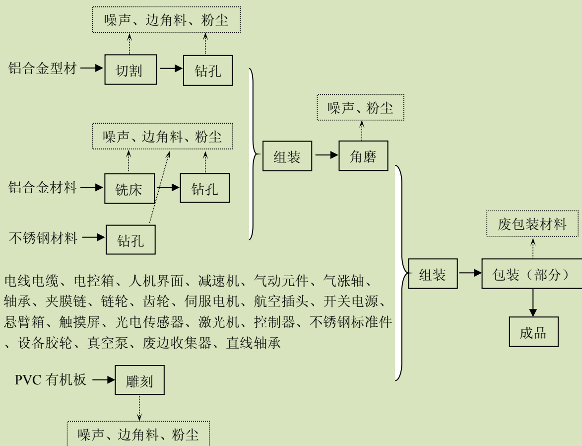
图 5-1 包装专用设备的制造工艺流程及产污点图
