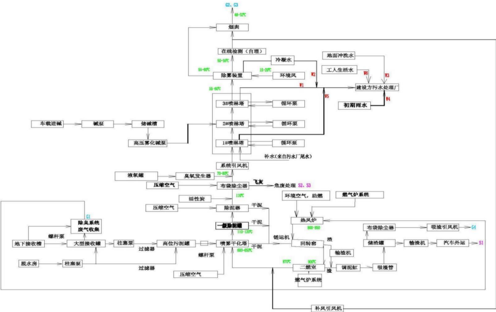
图 3.1-1 现有项目工艺流程图
