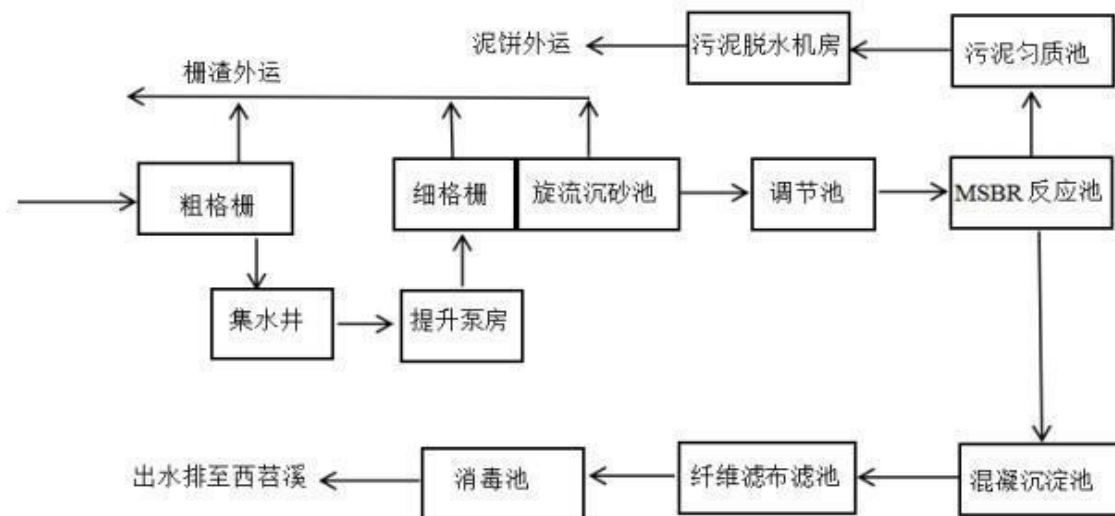
图 4.3-2 安吉净源污水处理有限公司安吉城北污水处理厂三期处理工艺流程图
