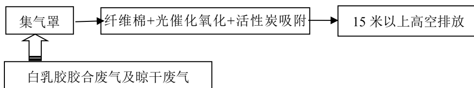
图 5-4 废气处理流程图
