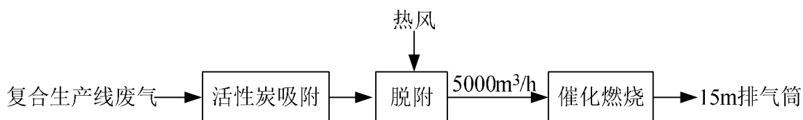
图 8-1 废气处理工艺流程图
