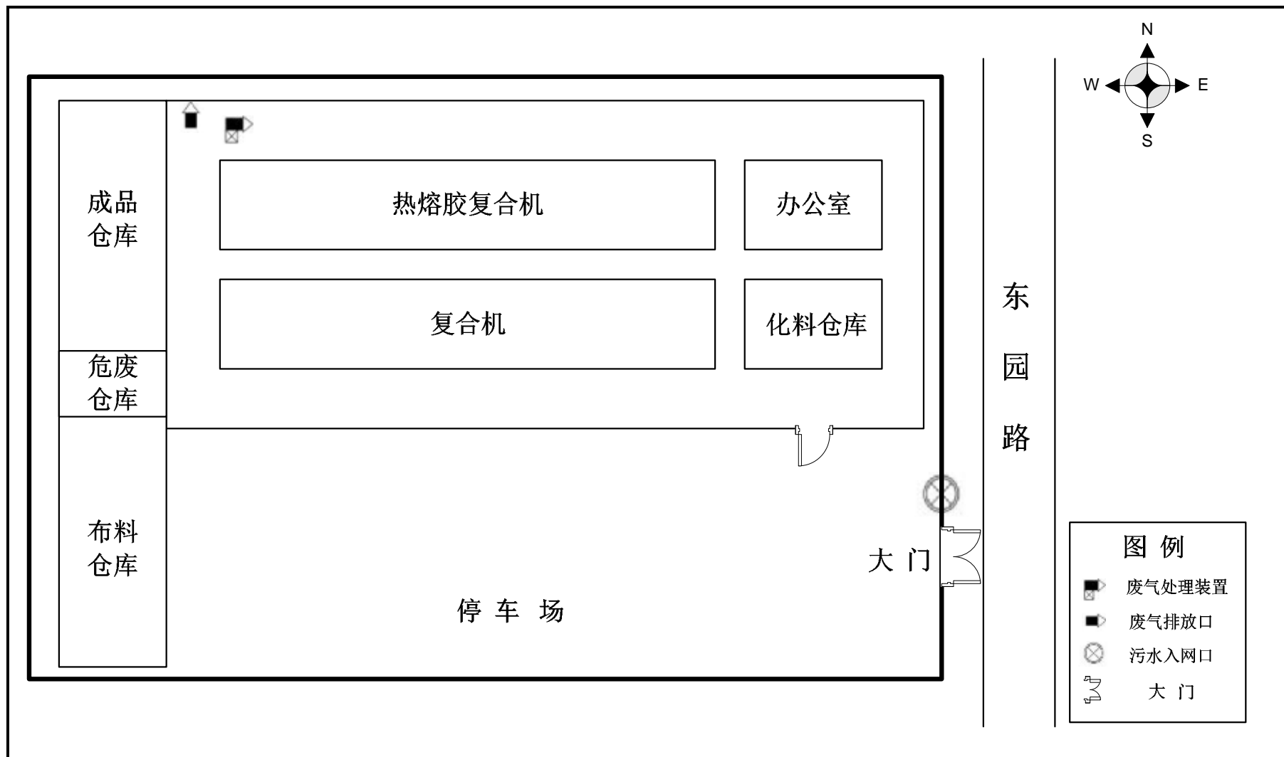
附图2 厂区总平布置图
