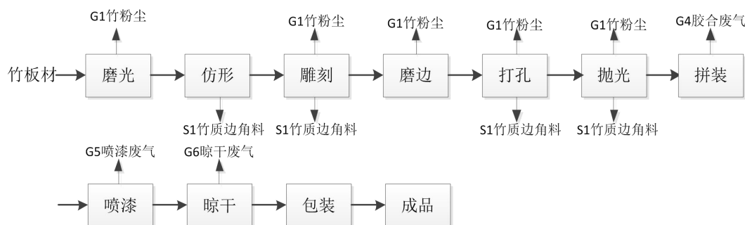
图 5-2 项目竹小家具生产工艺流程图
