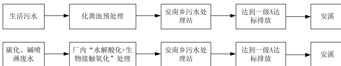
图 5-3 废水处理流程图
