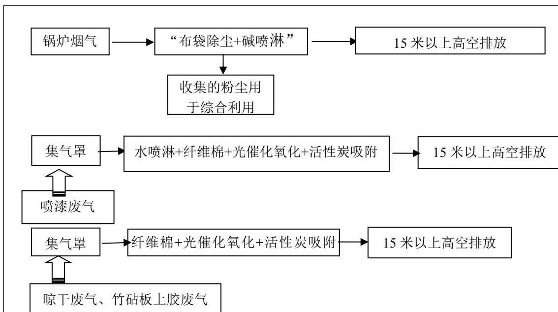
图 5-4 废气处理流程图
