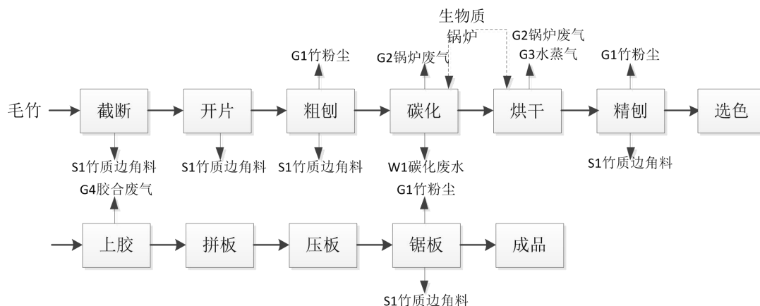
图 5-1 项目竹砧板生产工艺流程图
