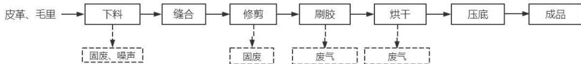
图 5-1 项目工艺流程及产污环节图
