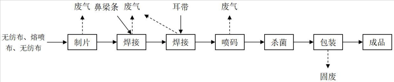
图 5-1 生产工艺 1 流程图
