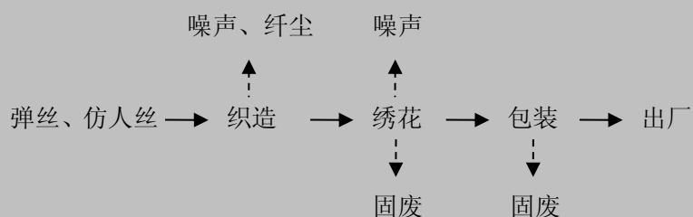
图 1-1 装饰布生产工艺流程图
