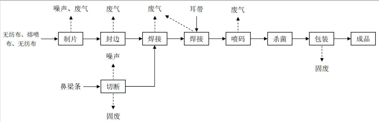
图 5-2 生产工艺 2 流程图
