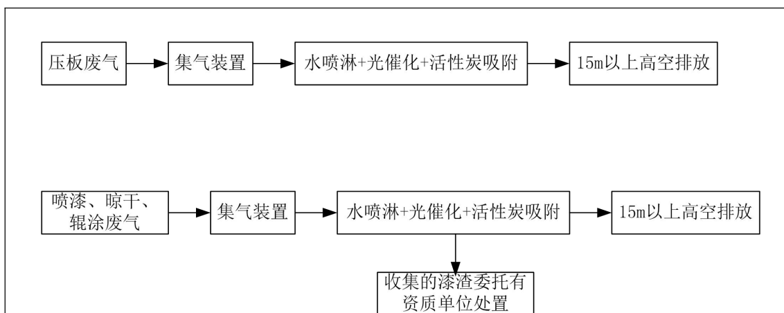
图 5-3 废气处理流程图
