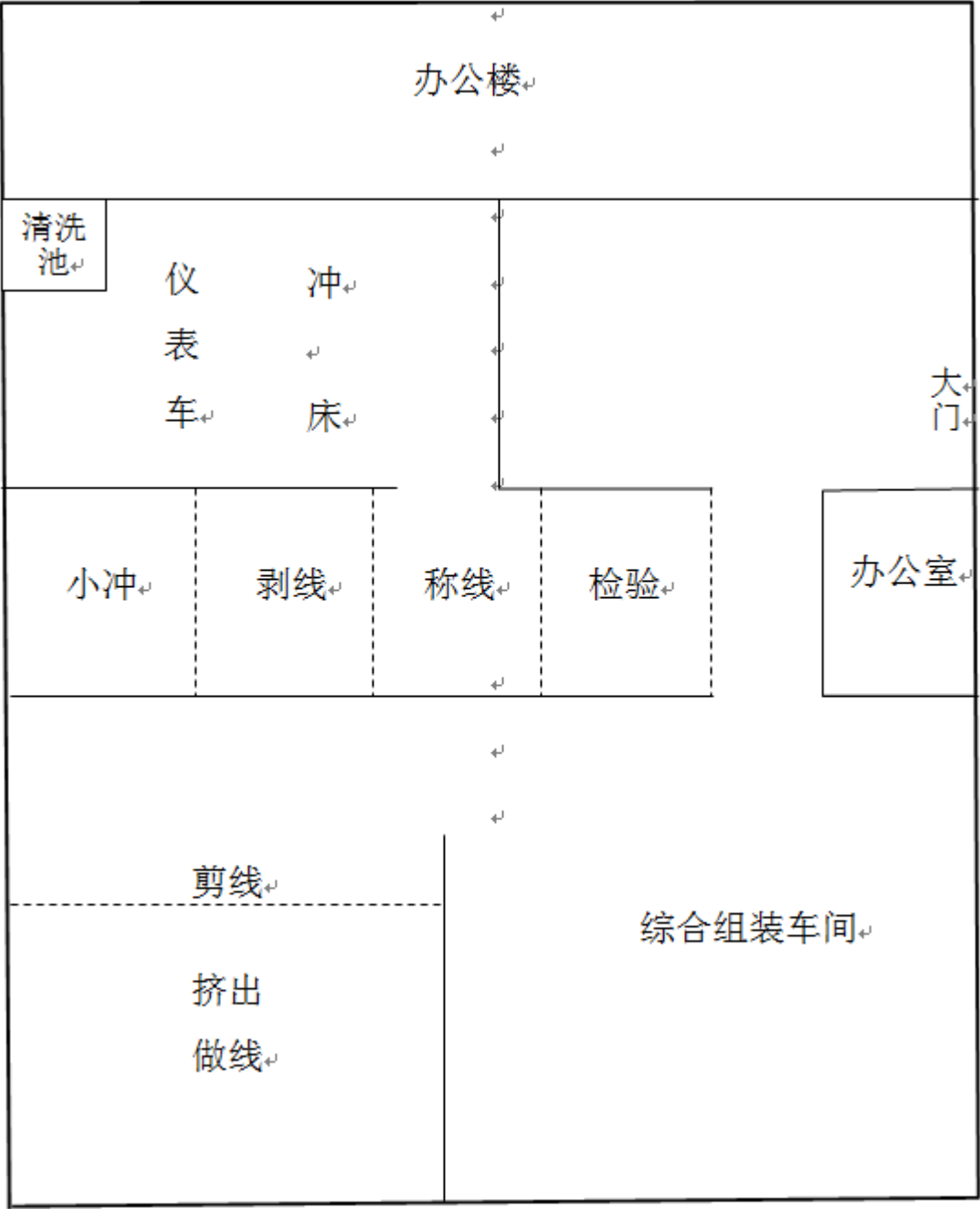
图 3.2-1 项目厂区总平面布局
