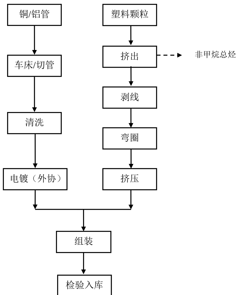
图 3.5-1 本项目超市防盗绳工艺流程图
