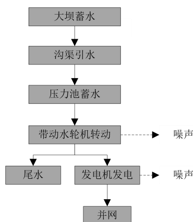
图 3-3 生产工艺流程图
