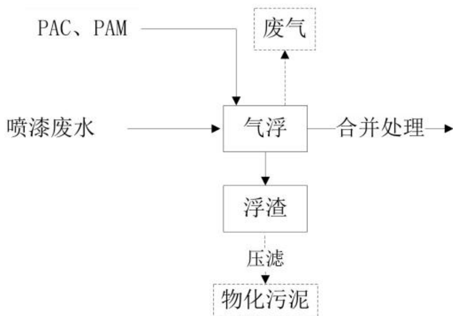
图 4-5 喷漆废水预处理工艺流程图
