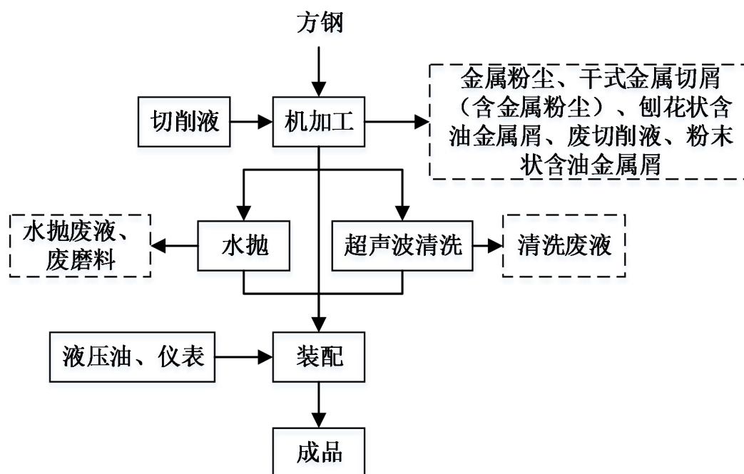
图 2-2 生产工艺流程及产污节点图 (生产过程均有不同程度噪声产生)
