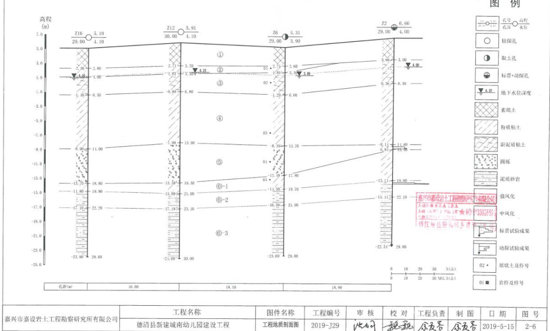
图 3-3 场地内工程地质剖面图
