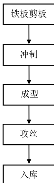
图 3.5-1 本项目锁体配件工艺流程图
