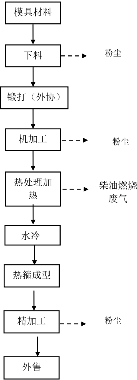
图 3.5-1 本项目模具精板工艺流程图
