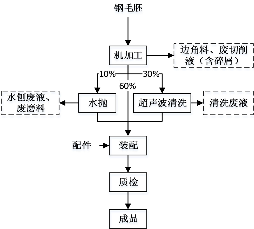
图 2-2 生产工艺流程及产污节点图
