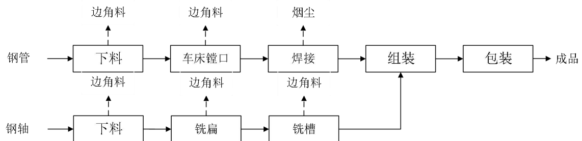
图 5-3 滚筒生产工艺流程图
