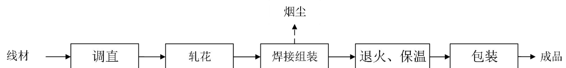
图 5-2 合金焊接筛网生产工艺流程图
