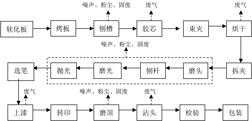
图 5-2 铅笔生产工艺
