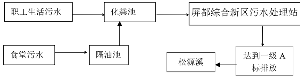
图 5-2 废水处理流程图
