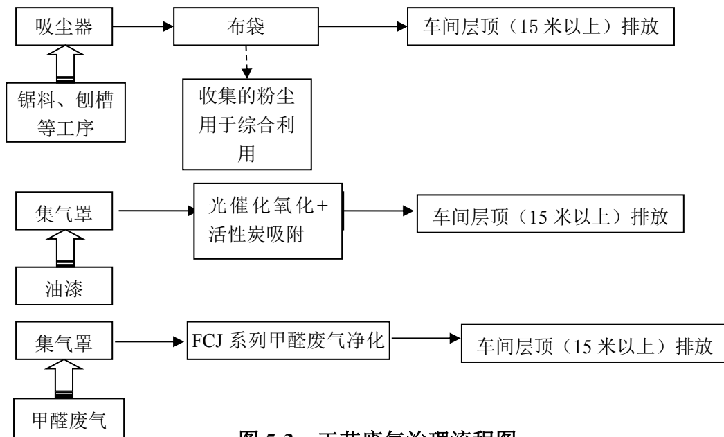
图 5-3 工艺废气治理流程图
